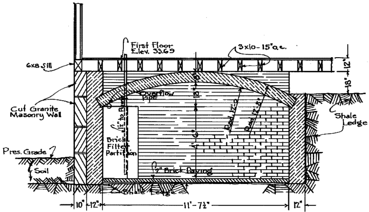
SECTION A-A
